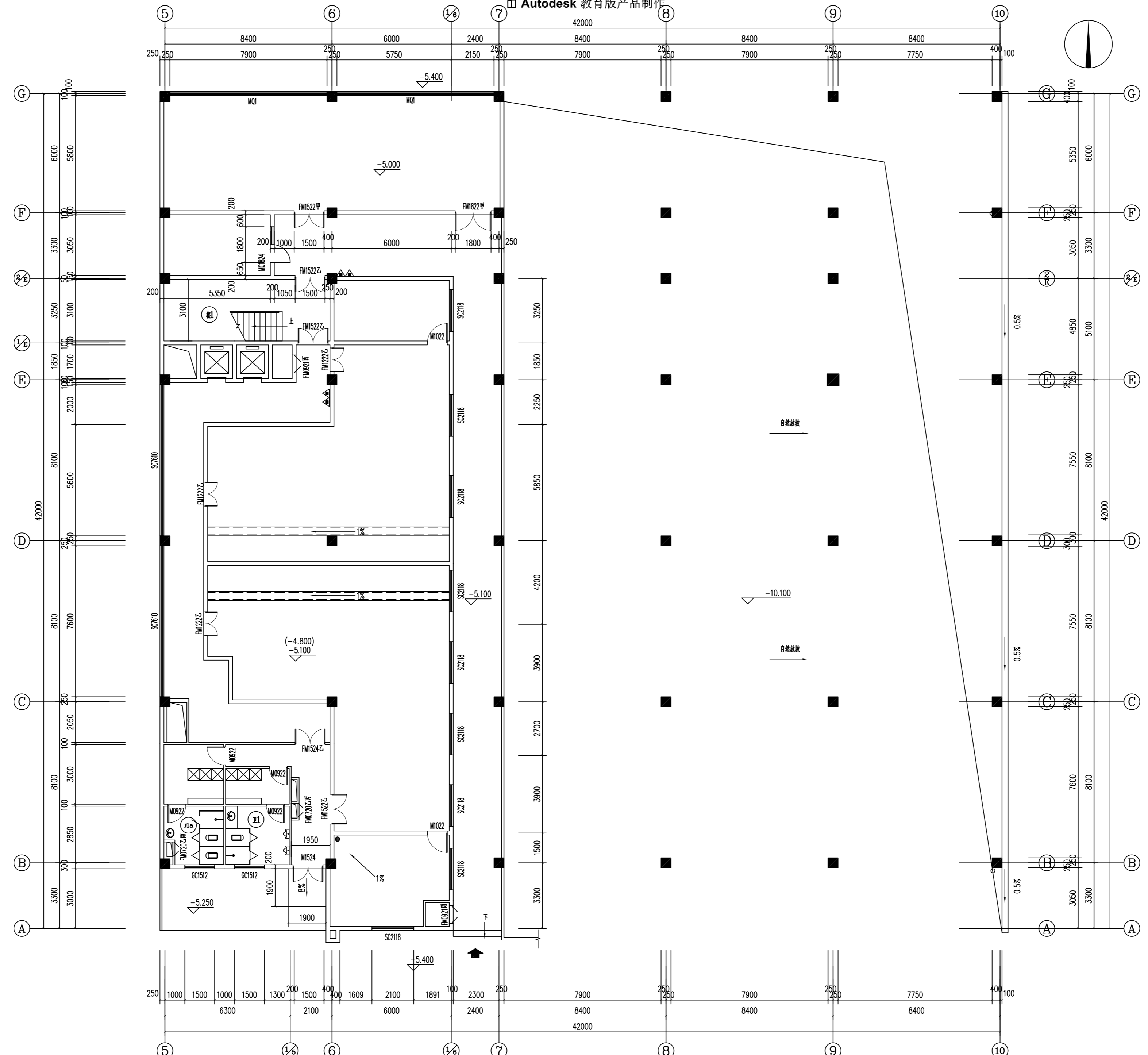
食堂及文体用房负一层平面 1:100
